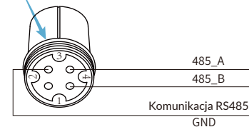
Rys. 7.6 Schemat połączeń licznika Eastron
