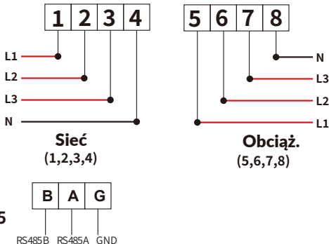
Rys. 7.18 Licznik Eastron
