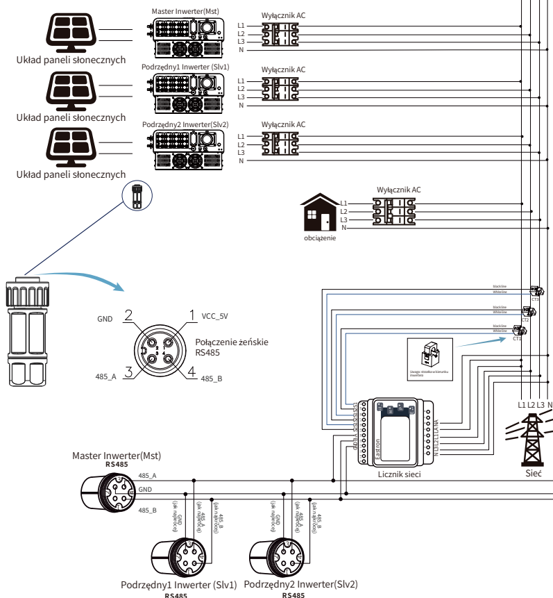
Rys. 7.23 Schemat połączeń (prąd trójfazowy)
