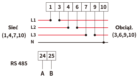
Rys. 7.11 Licznik CHINT
