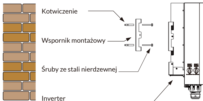
Rys. 4.4 Instalacja inwertera
