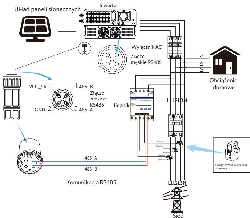
Rys. 7.14 Schemat połączeń licznika CHINT
