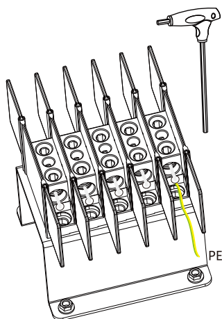
Rys 5.11 The Instalacja przewodu uziemienia obudowy
