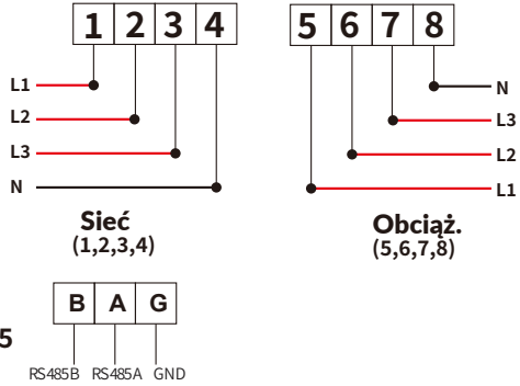
Rys. 7.20 Licznik Eastron
