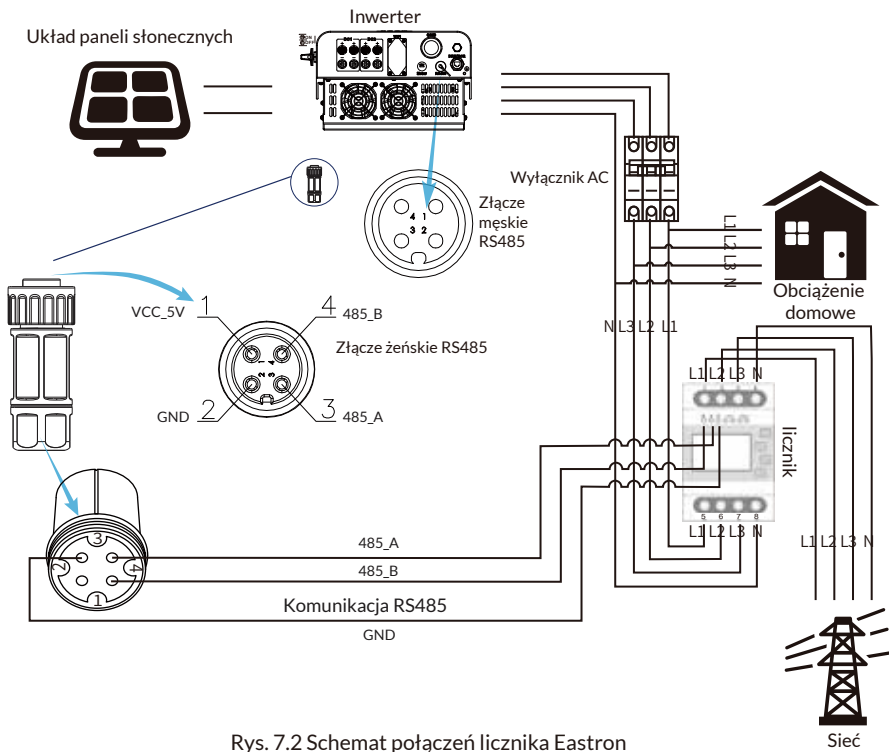
Rys. 7.2 Schemat połączeń licznika Eastron
