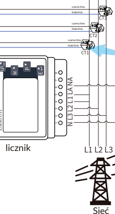
Rys. 7.6 Schemat połączeń licznika Eastron
