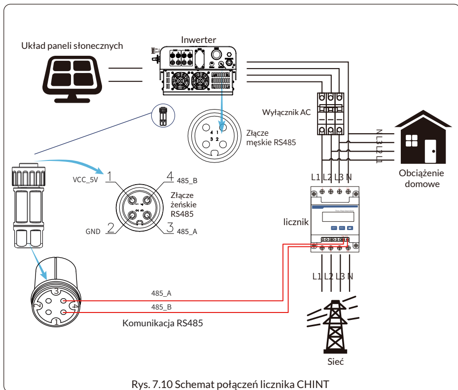
Rys. 7.10 Schemat połączeń licznika CHINT
