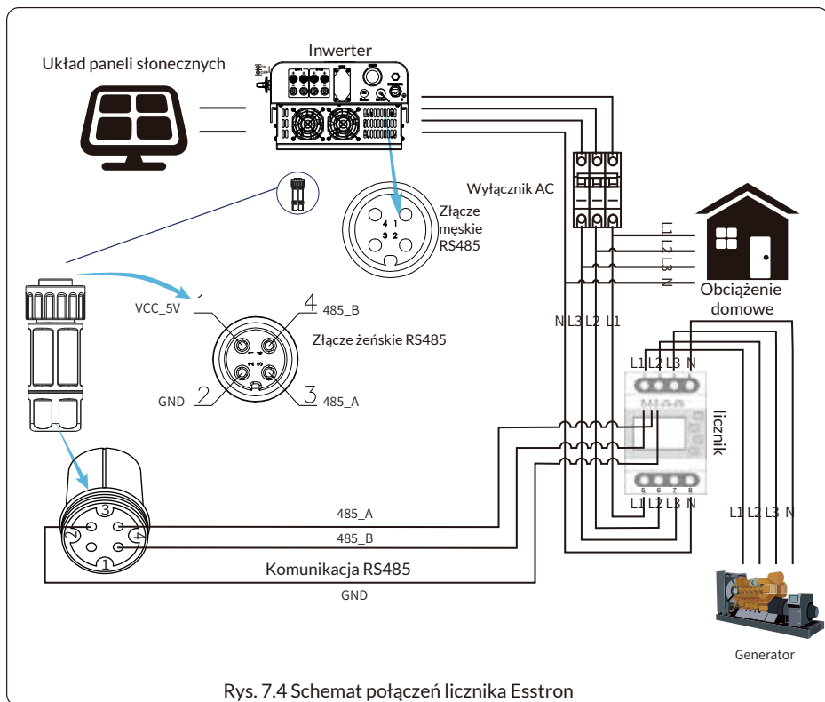
Rys. 7.4 Schemat połączeń licznika Esstron
