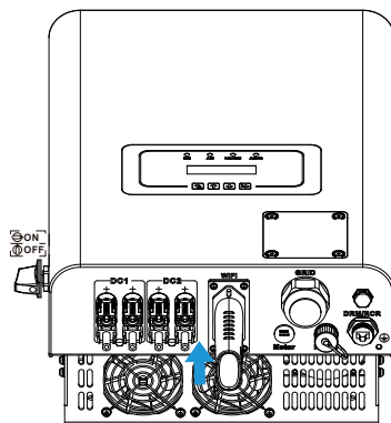
Rys. 5.13 Schemat instalacji rejestratora danych
