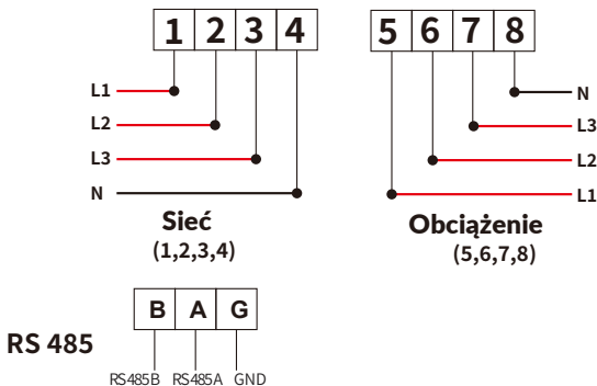
Rys. 7.3 Licznik Eastron
