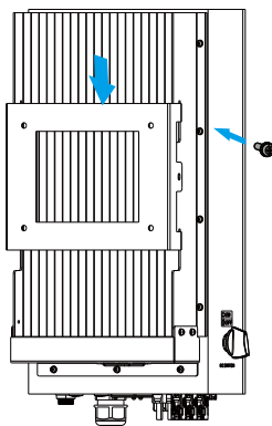
Rys. 4.6 Instalacja inwertera
