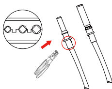
Rys. 5.4 Zaciśnięcie styku do przewodu
