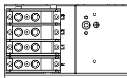
Rys. 5.10 Dokręcanie kabla połączeniowego AC
