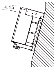
Rys. 4.2 Kąt instalacji
