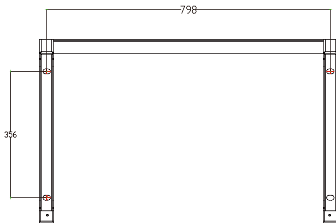
Rys. 4.4 Wymiary wspornika montażowego
