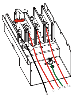
Rys. 5.9 Kabel AC podłączony do zacisku
