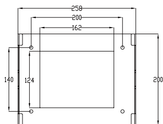
Rys. 4.5 Montaż płyty do zawieszania inwertera
