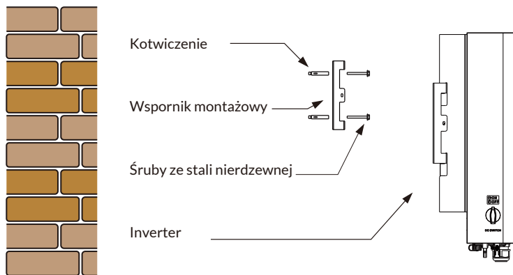
Rys. 4.4 Instalacja inwertera
