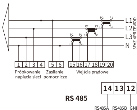
Rys. 7.7 Licznik Eastron
