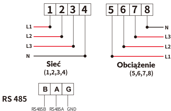
Rys. 7.3 Licznik Eastron
