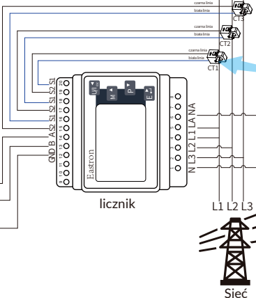
Rys. 7.6 Schemat połączeń licznika Eastron
