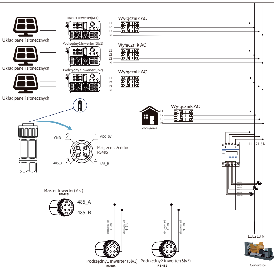
Rys. 7.33 Schemat połączenia CHINT (tabela przelotowa)
