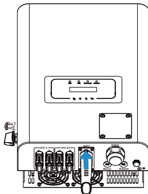
Rys. 5.13 Schemat instalacji rejestratora danych
