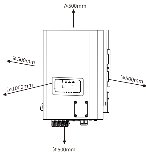
Rys. 4.3 Szczelina instalacyjna
