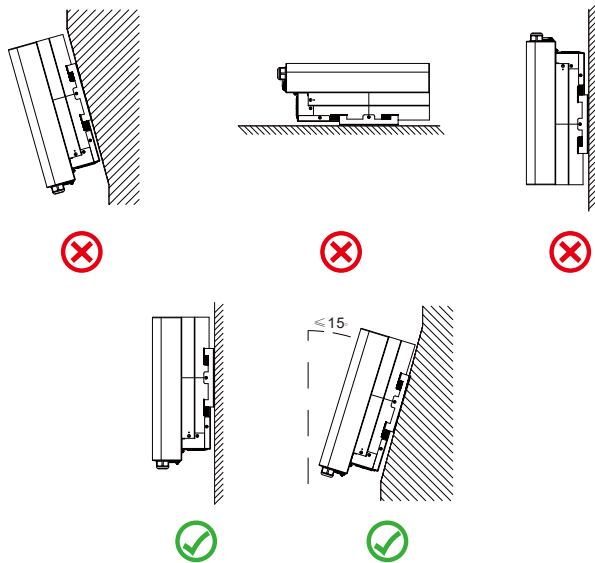
Rys. 4.2 Kąt instalacji
