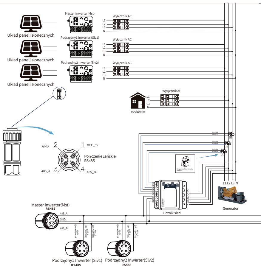
Rys. 7.25 Schemat połączeń (prąd trójfazowy)
