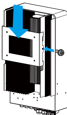
Instalacja płyty do zawieszania inwertera
