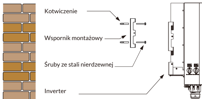
Rys. 4.4 Instalacja inwertera
