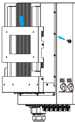
Rys. 4.6 Instalacja inwertera
