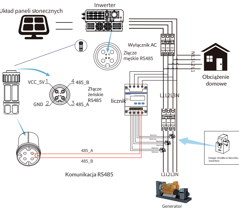
Rys. 7.16 Schemat połączeń licznika CHINT
