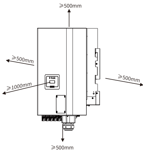
Rys. 4.3 Szczelina instalacyjna
