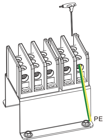
Rys 5.11 The Instalacja przewodu uziemienia obudowy
