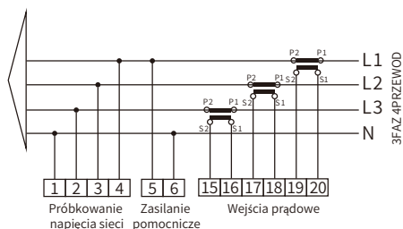
Rys. 7.22 Licznik Eastron
