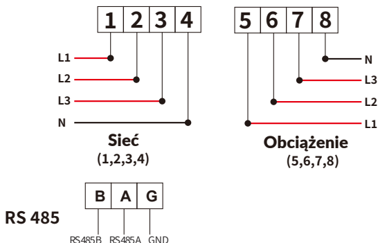
Rys. 7.1 Licznik Eastron
