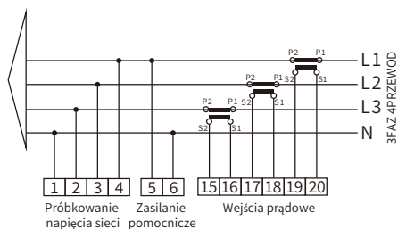
Rys. 7.24 Licznik Eastron
