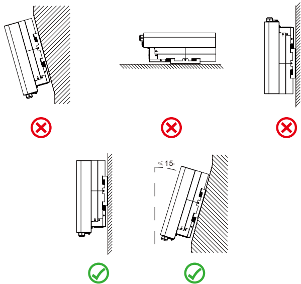
Rys. 4.2 Kąt instalacji
