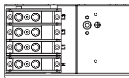
Rys. 5.10 Dokręcanie kabla połączeniowego AC
