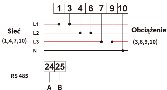
Rys. 7.11 Licznik CHINT
