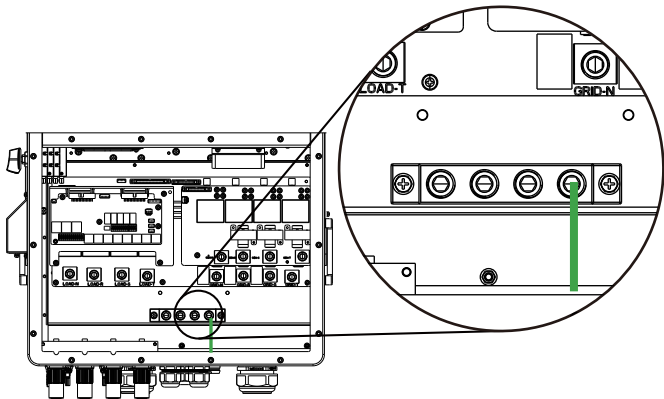
Podłączenie uziemienia (przewody miedziane) (obejście)
