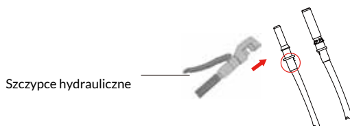
Rys. 5.4 Zaciśkanie styku do przewodu
