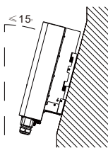
Rys. 4.2 Kąt instalacji
