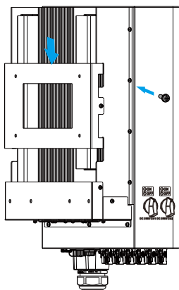
Rys. 4.6 Instalacja inwertera
