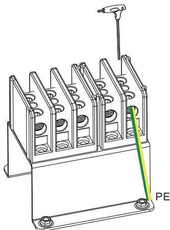
Rys 5.11 The Instalacja przewodu uziemienia obudowy
