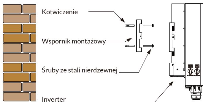
Rys. 4.4 Instalacja inwertera
