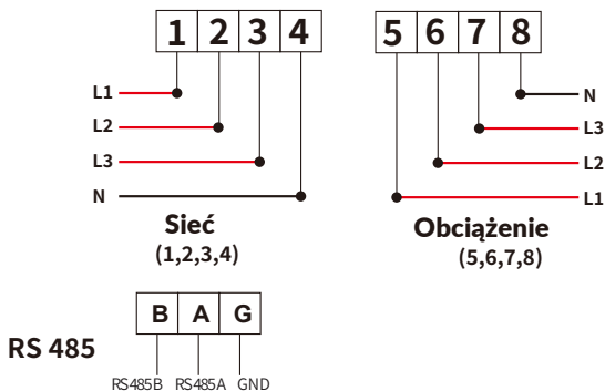
Rys. 7.3 Licznik Eastron
