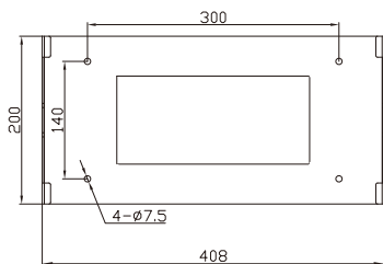
Rys. 4.5 Montaż płyty do zawieszania inwertera
