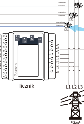
Rys. 7.6 Schemat połączeń licznika Eastron
