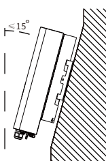
Rys. 4.2 Kąt instalacji
