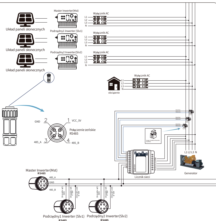
Rys. 7.24 Licznik Eastron
