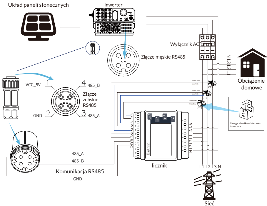
Rys. 7.6 Schemat połączeń licznika Eastron
