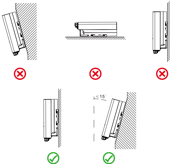
Rys. 4.2 Kąt instalacji
