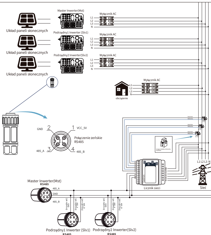
Rys. 7.23 Schemat połączeń (prąd trójfazowy)
