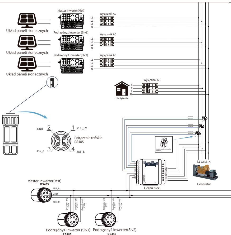
Rys. 7.25 Schemat połączeń (prąd trójfazowy)
