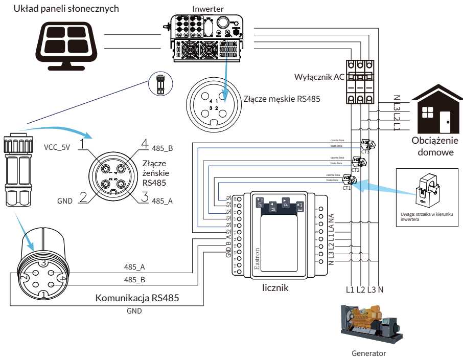
Rys. 7.8 Schemat połączeń licznika Eastron
