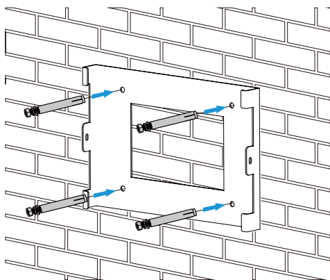
Rys. 4.5 Montaż płyty do zawieszania inwertera
