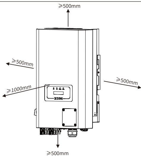
Rys. 4.3 Szczelina instalacyjna
