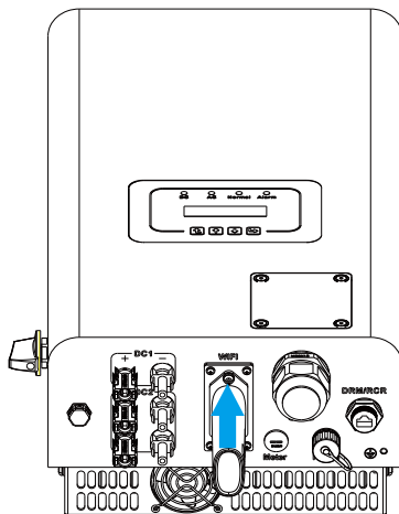
Rys. 5.10 Schemat instalacji rejestratora danych
