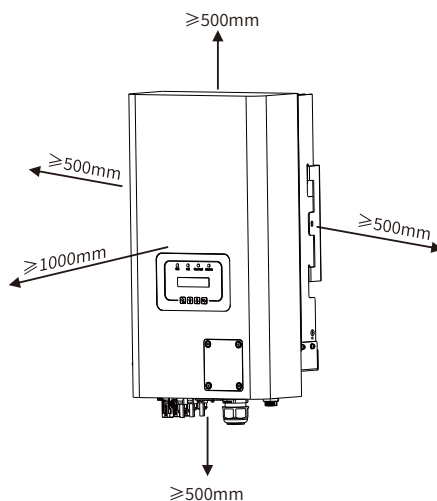
Rys. 4.3 Szczelina instalacyjna
