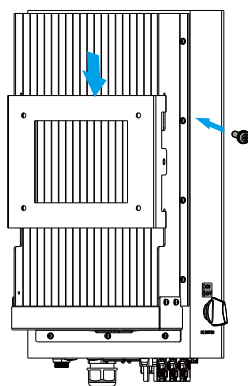
Rys. 4.6 Instalacja inwertera
