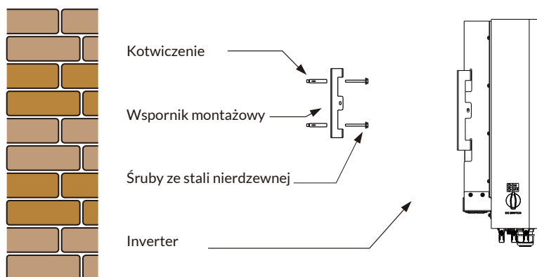
Rys. 4.4 Instalacja inwertera
