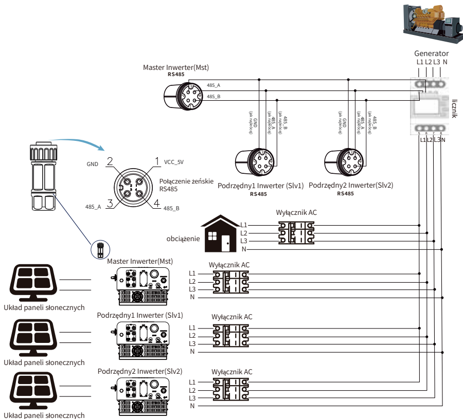
Rys. 7.21 Schemat połączeń Eastron (tabela przelotowa)
