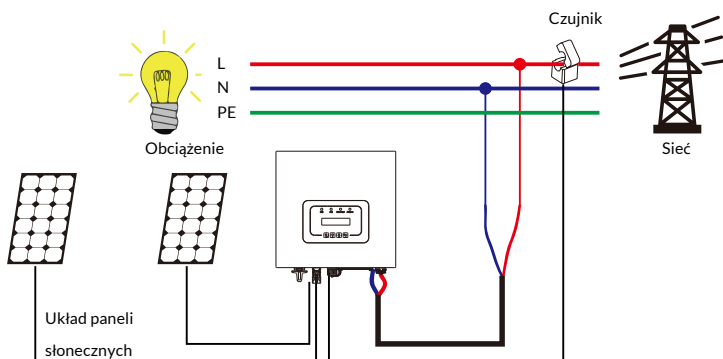
Rys. 7.23 Schemat połączeń zacisku czujnika
