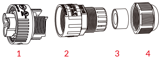
1. Gniazdo 2.Tuleja 3.Rdzeń uszczelniający 4.Nakrętka uszczelniająca
