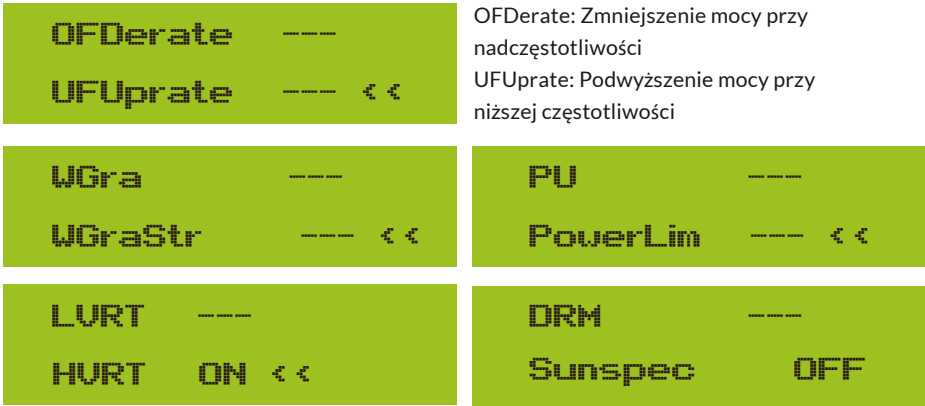
Rys. 8.33 Spadek mocy czynnej
