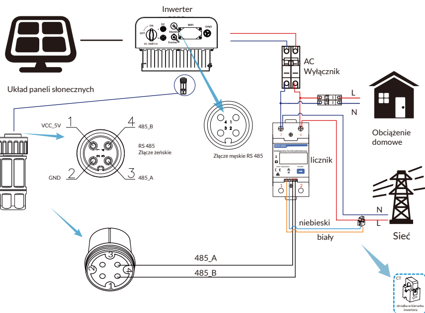
Rys. 7.9 Licznik CHNT
