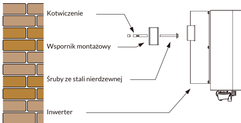
Rys. 4.4 Instalacja inwertera
