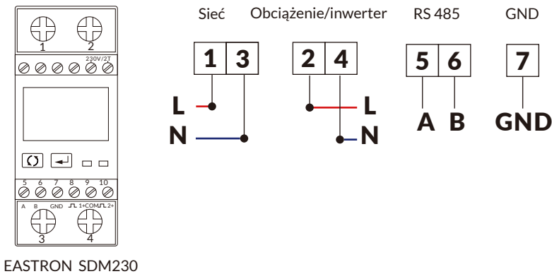
Rys. 7.11 Licznik EASTRON
