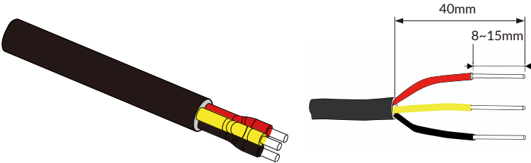
Rys. 5.8 Ściągania izolacji kabla AC
