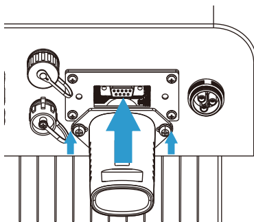
Rys. 5.13 Schemat instalacji rejestratora
