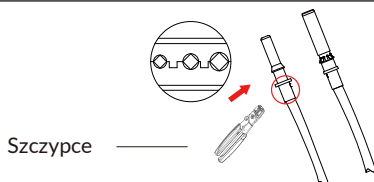
Rys. 5.4 Zaczepianie styku do przewodu
