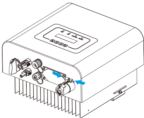
Rys. 5.15 Dodaj jednofazową tuleję ochronną
