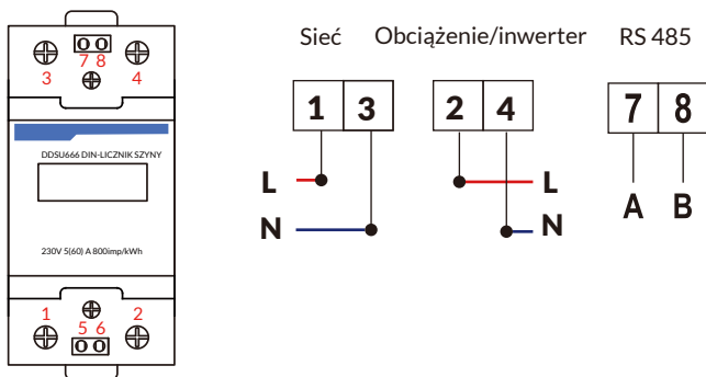
CHNT DDSU666
