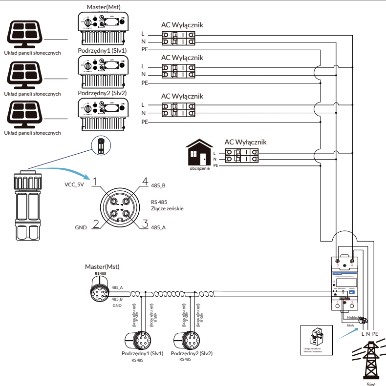
Rys. 7.17 Licznik CHNT
