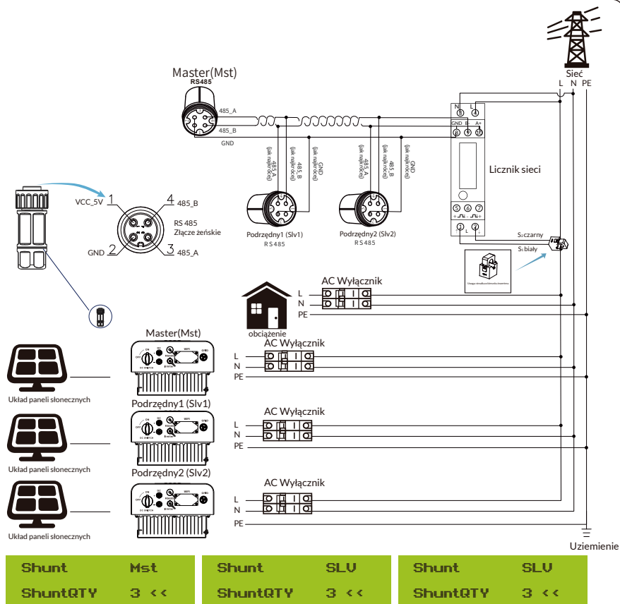
Rys. 7.14 Schemat połączeń Easton (tabela przelotowa)
