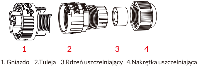
Rys. 5.7 Struktura złącza AC
