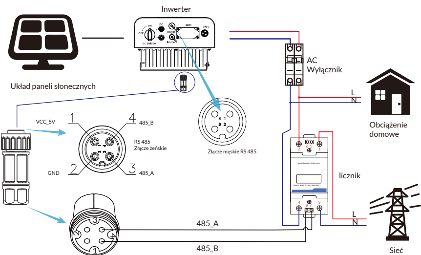
Rys. 7.7 Schemat połączeń licznika CHNT
