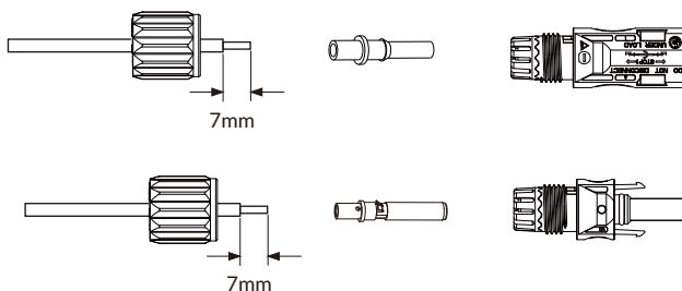
Rys. 5.3 Demontaż nakrętki zasłaniającej złącza
