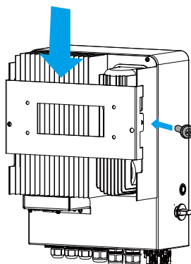
Instalacja płyty do zawieszania inwertera
