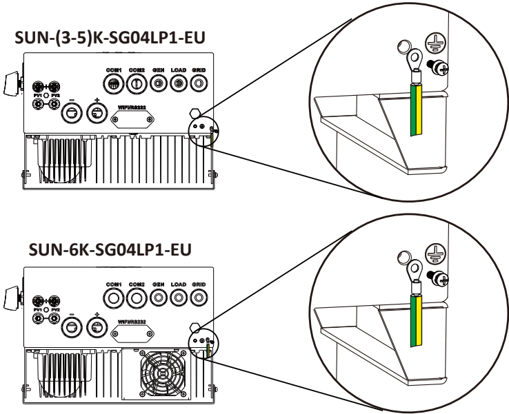
Podłączenie uziemienia (przewody miedziane)
