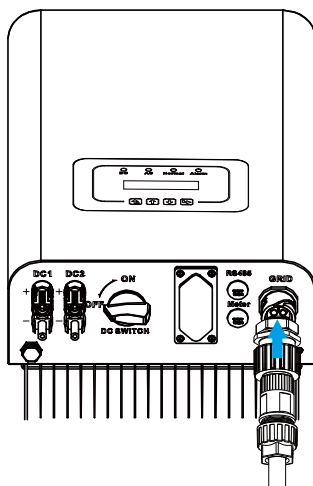
Abb. 5.10 AC-Eingangsanschluss
