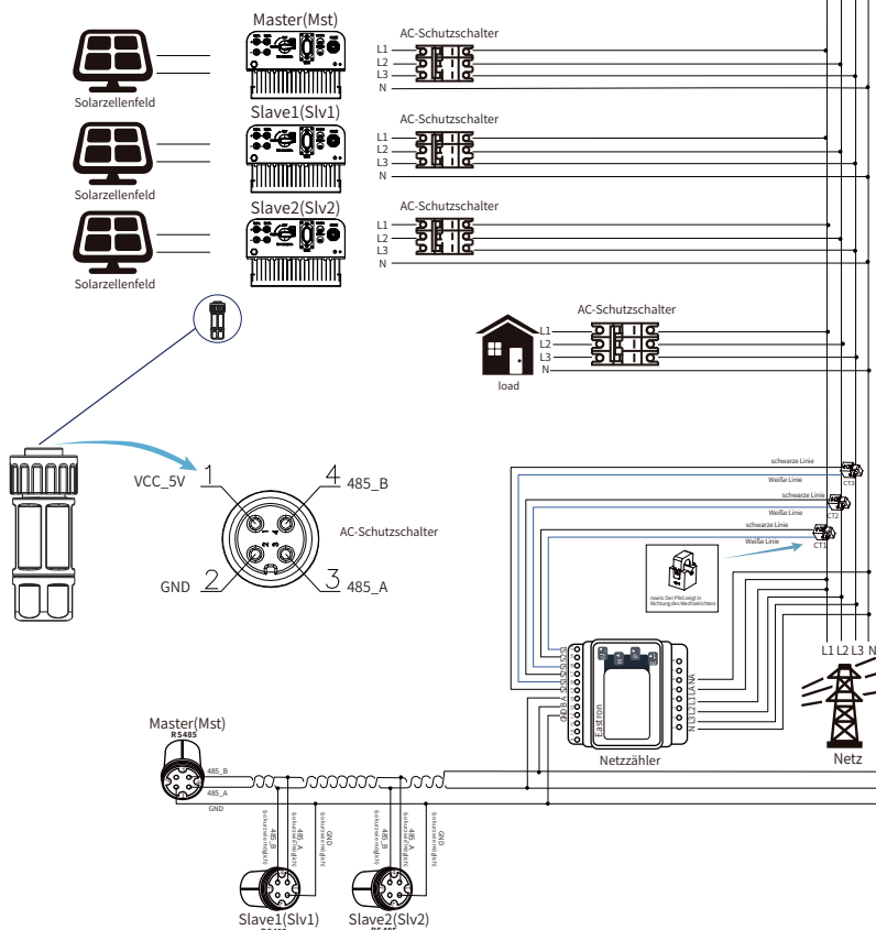
Abb. 7.23 Anschlussplan (Dreiphasenstrom)
