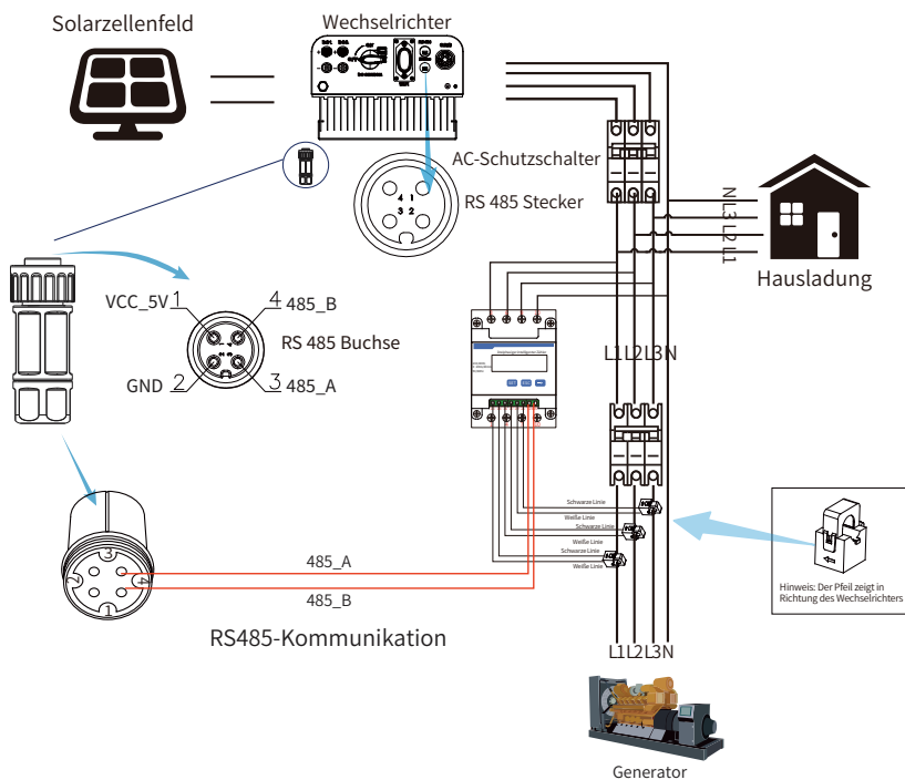
Abb. 7.16 Anschlussplan des CHINT-Zählers
