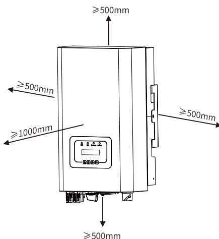
Abb. 4.3 Einbaulücke
