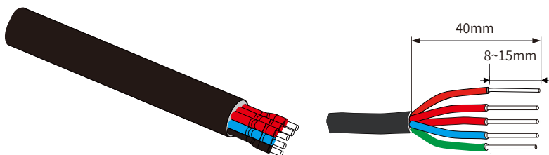
Abb. 5.8 AC-Kabel abisolieren
