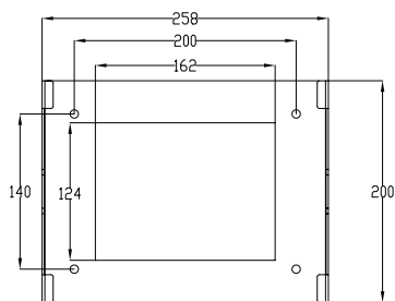
Abb. 4.5 Montage der Aufhängeplatte des Wechselrichters
