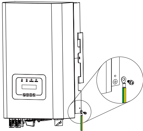
Abb. 5.12 Installation des Mantelerdungsdrahtes
