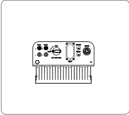
Abb. 1.2 Ansicht von unten
