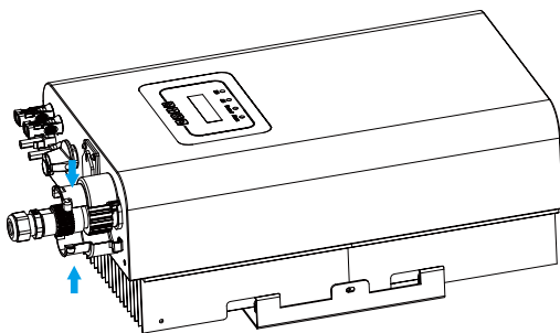
Abb. 5.11 Fügen Sie eine dreiphasige Schutzhülle für
