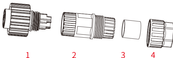
1. Passende Muffe 2. Hülse 3. Dichtungskern 4. Dichtungsmutter
